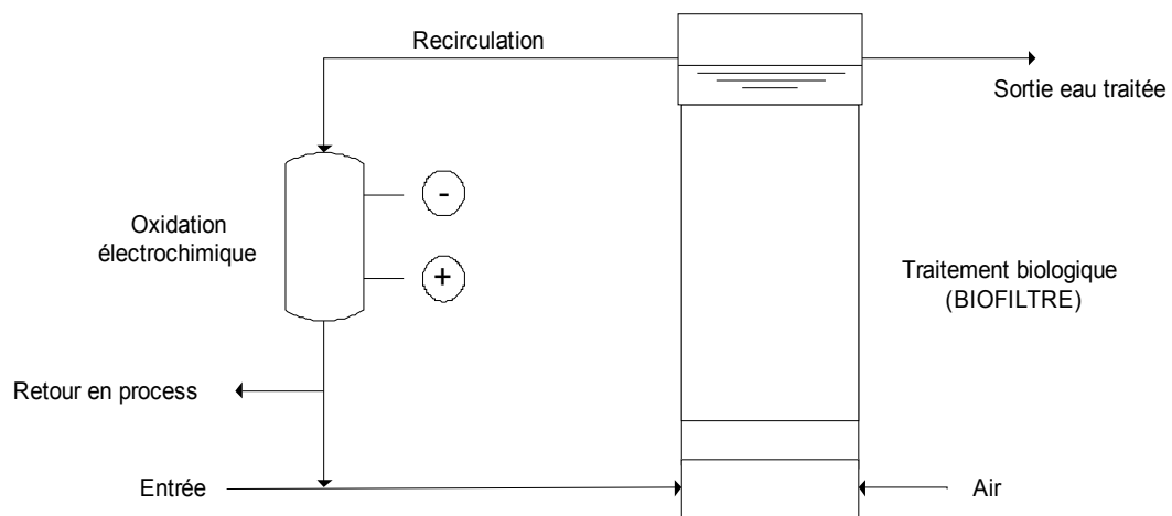
Image 1 : Schéma du procédé AQUA-BIOMANT
